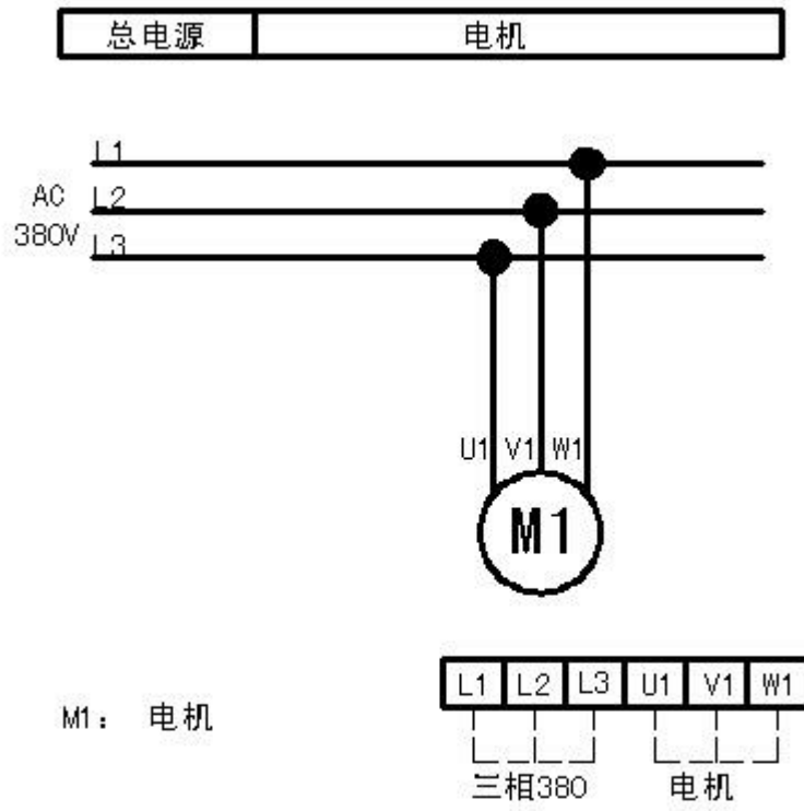
图二 总电路图
